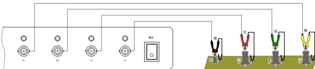
图 2 绕组接线图
