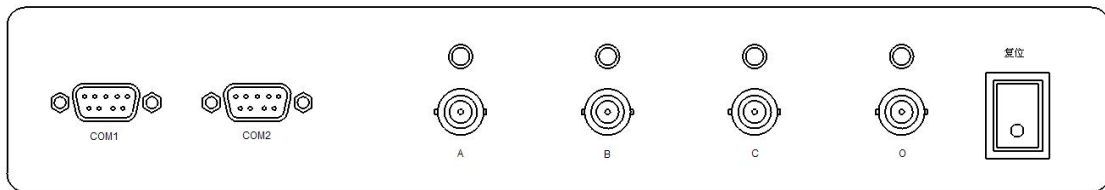
图 1b 变压器绕组变形测试仪后面板图（后面板）
