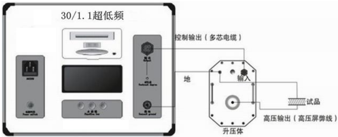
图 4a 30/1.1 或 50/1.1 (连接图)
