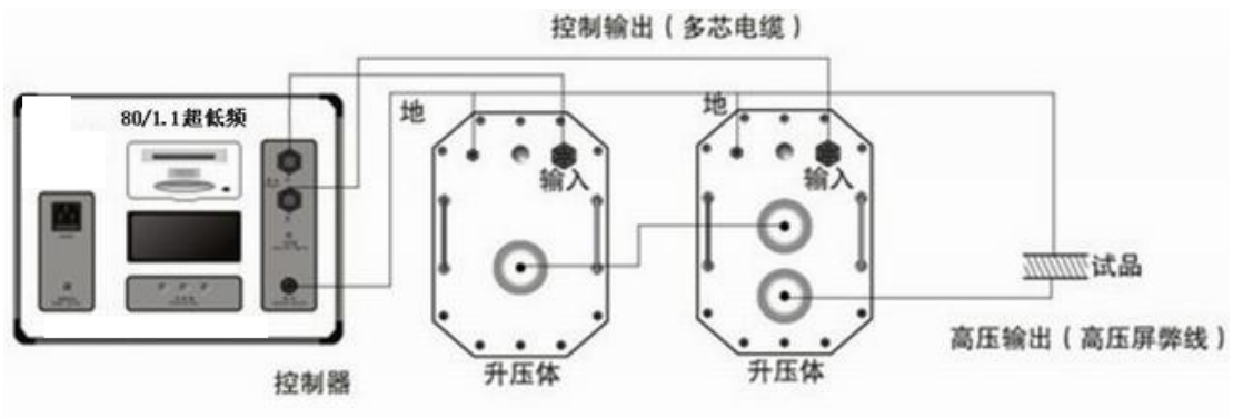
图 4b 80/1.1 (连线图)
